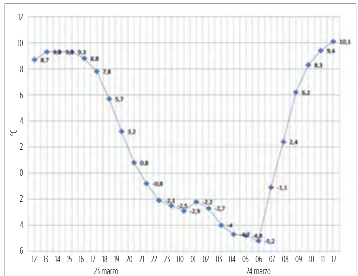
FIG. 3 TEMPERATURA 23-24 MARZO
