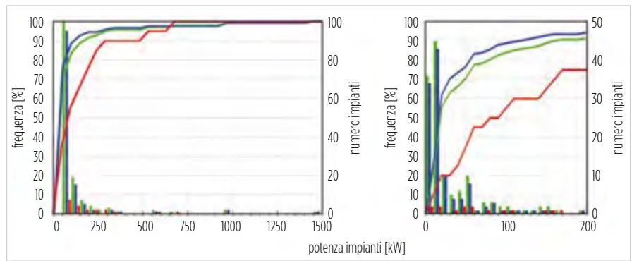
FIG. 3 POTENZA TERMICA
