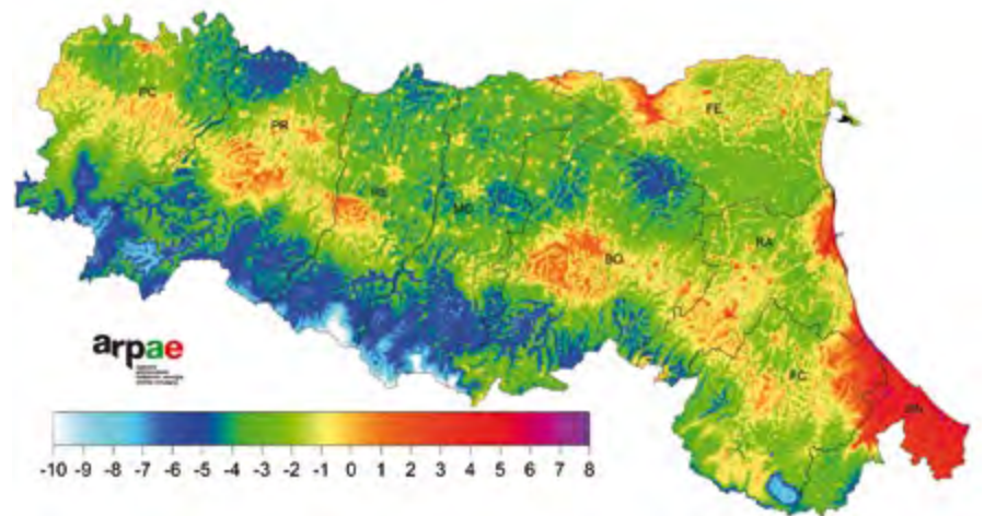
FIG. 4 TEMPERATURA 24 MARZO
