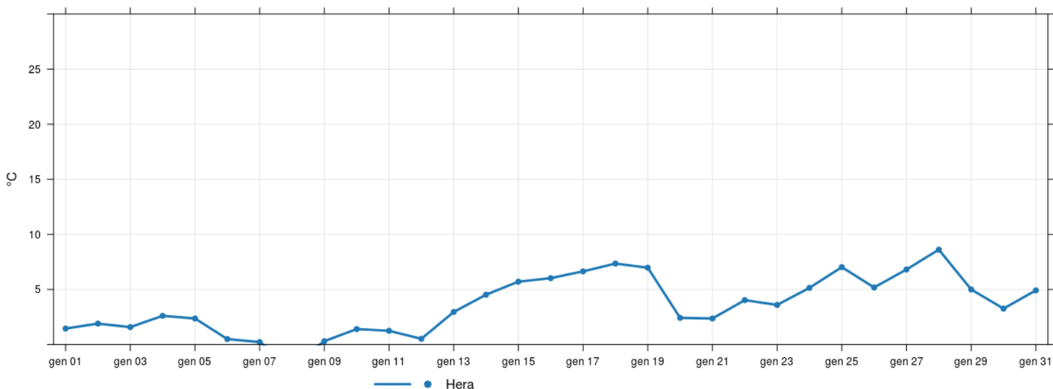
Temperatura media giornaliera
