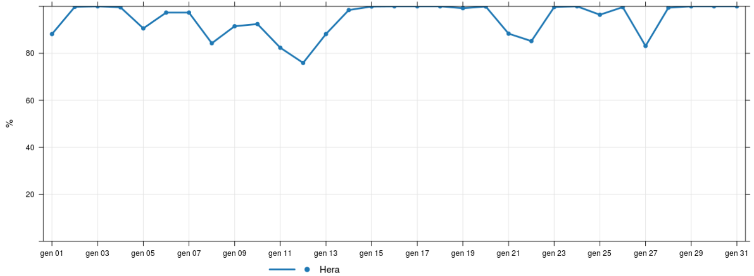
Figura 10:Umidità relativa media giornaliera
