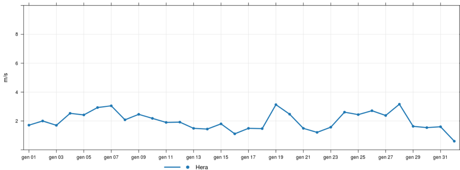
Figura 8: Velocità del vento – Massimi giornalieri
