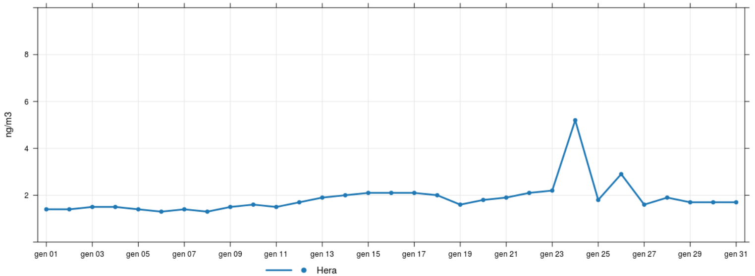
Mercurio - Massimi giornalieri
