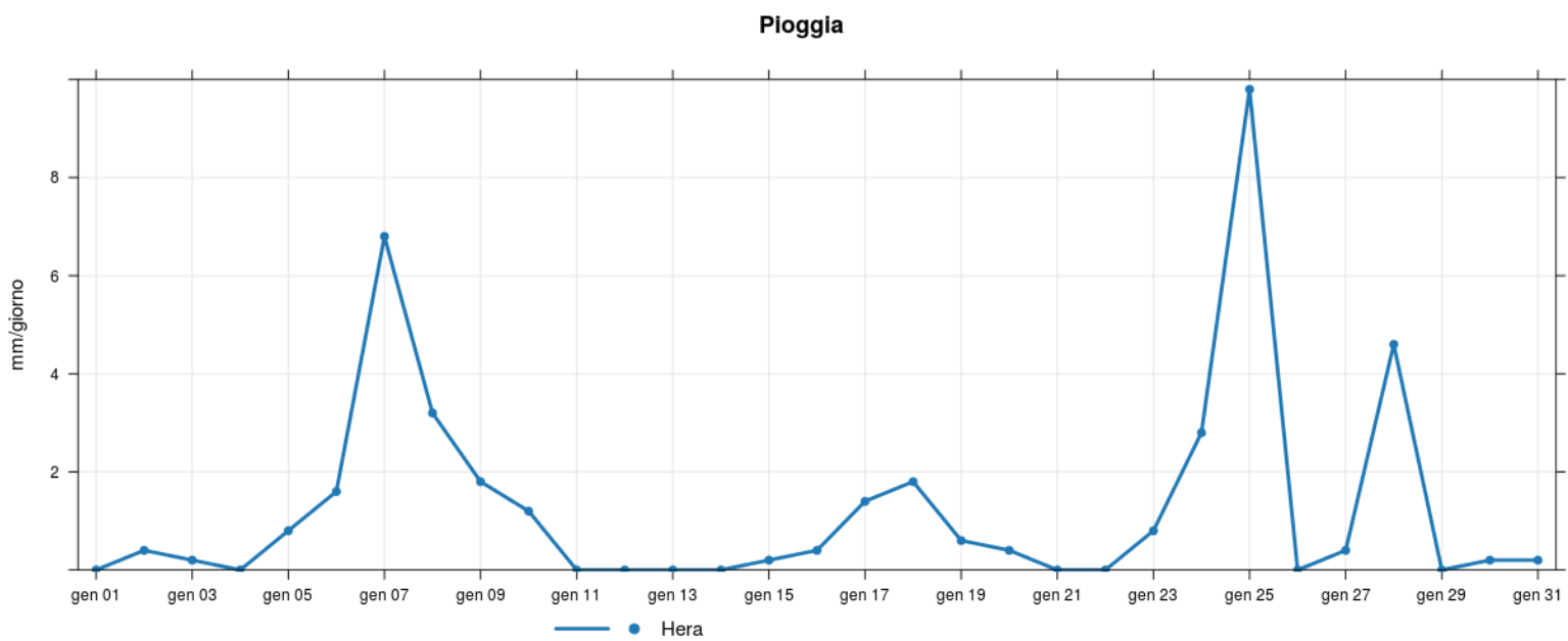
Figura 11:Pioggia cumulata nell'arco delle 24 ore
