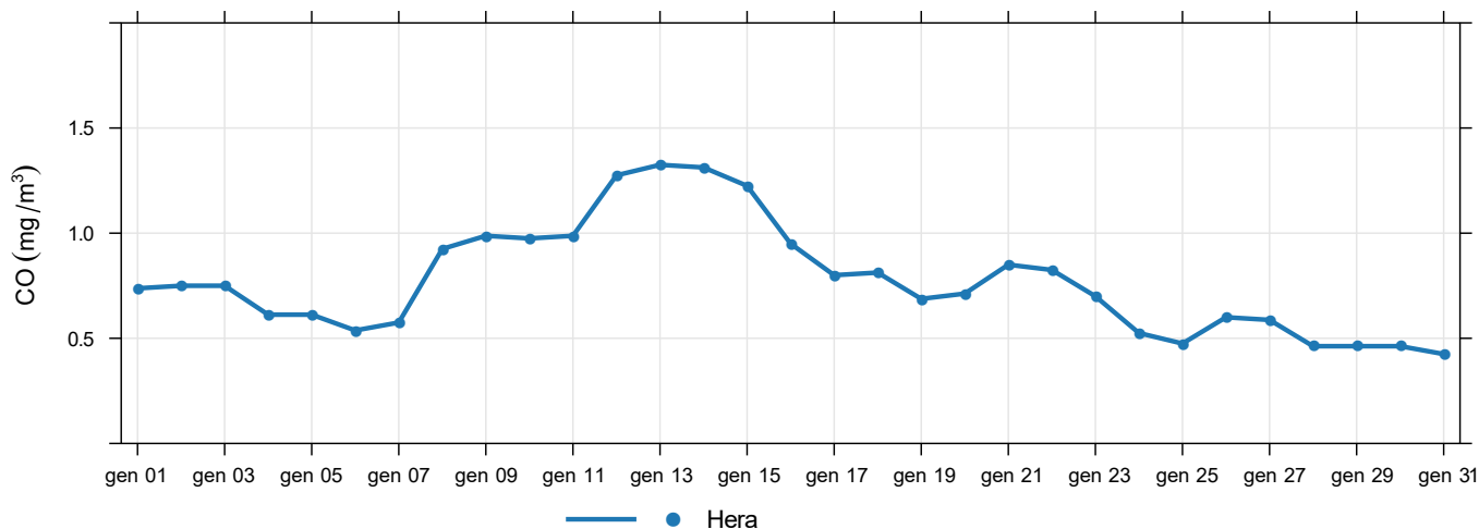
Figura 5: Massimi giornalieri della media di 8 ore di monossido di carbonio.
