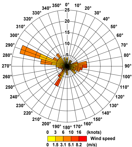
Velocità e direzione vento dal 17/8/07 al 23/8/07
