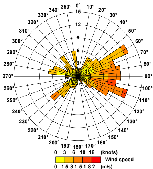
Velocità e direzione vento dal 11/9/07 al 17/9/07
