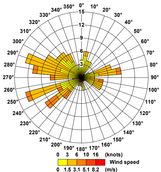
Velocità e direzione vento dal 10/1/07 al 16/1/07
