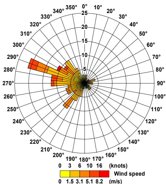
Velocità e direzione vento dal 4/12/07 al 10/12/07
