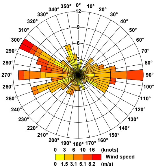
Velocità e direzione vento dal 13/2/07 al 19/2/07
