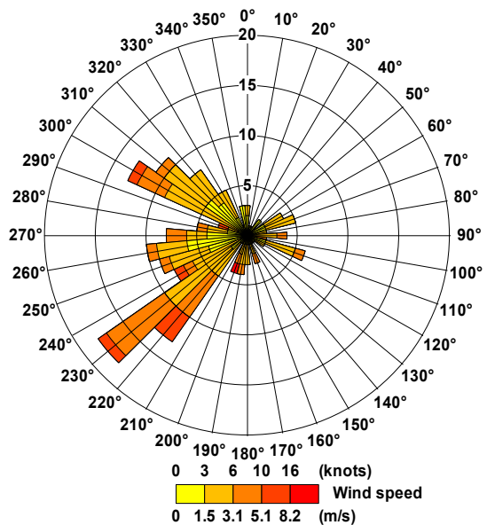
Velocità e direzione vento dal 13/3/07 al 19/3/07
