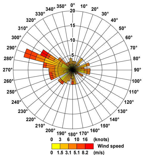
Velocità e direzione vento dal 10/5/07 al 16/5/07
