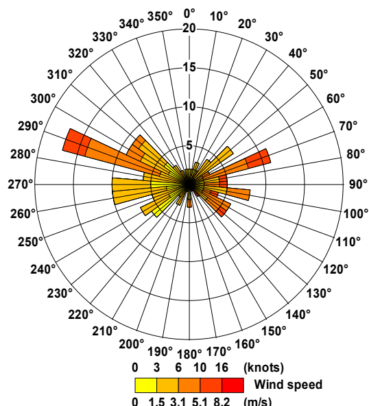
Velocità e direzione vento dal 16/10/07 al 22/10/07
