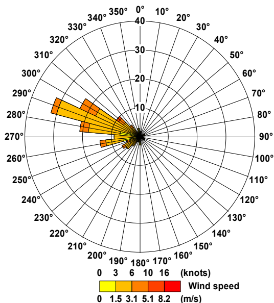
Velocità e direzione vento dal 13/11/07 al 19/11/07
