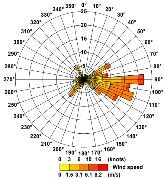
Velocità e direzione vento dal 20/4/07 al 26/4/07
