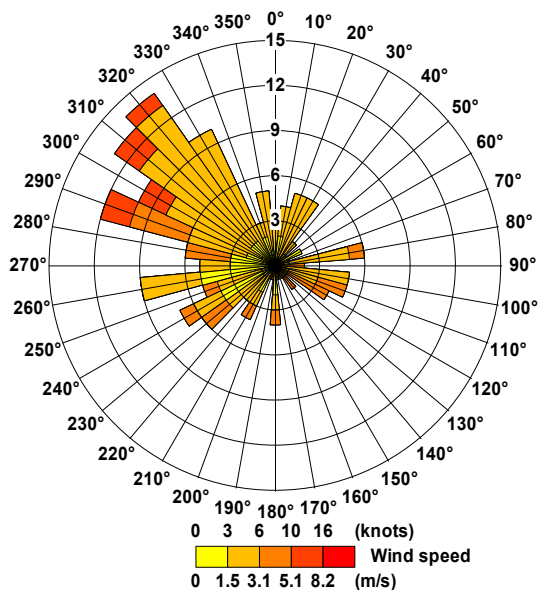
Velocità e direzione vento dal 10/7/07 al 16/7/07
