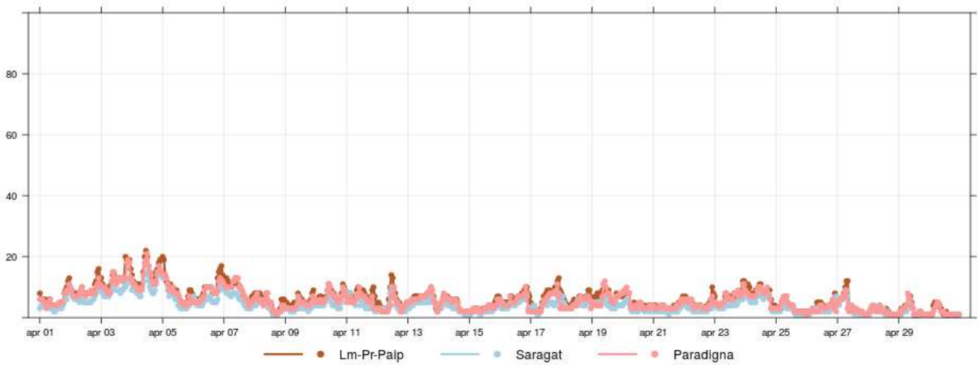
Figura 10: PM1, andamento orario giornaliero.
