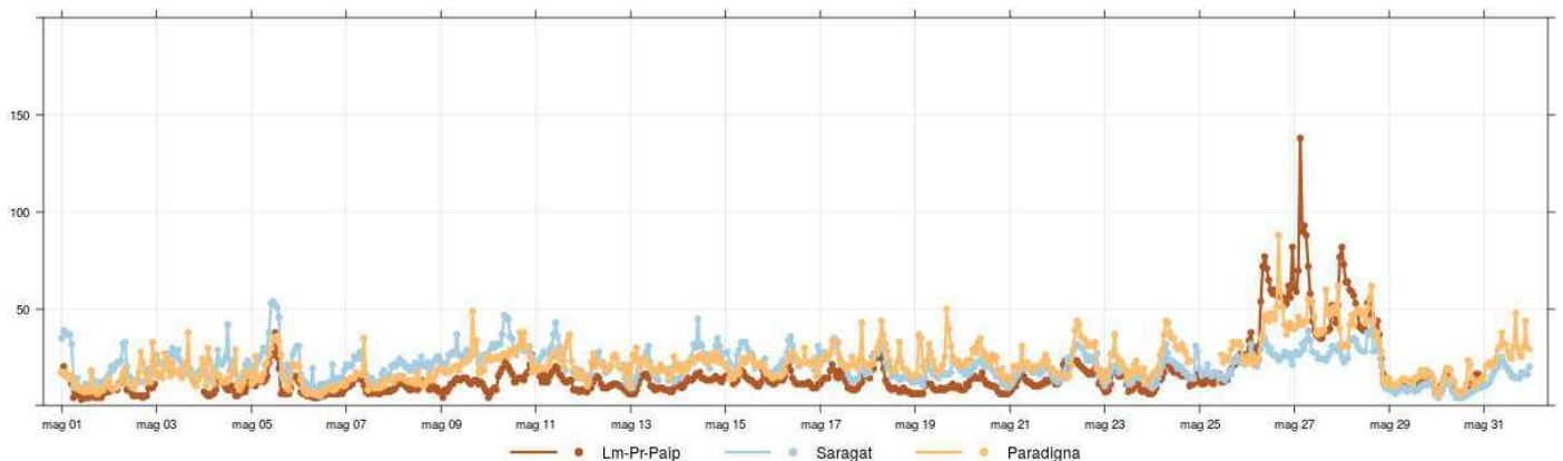
Figura 12: PM10, andamento orario giornaliero.
