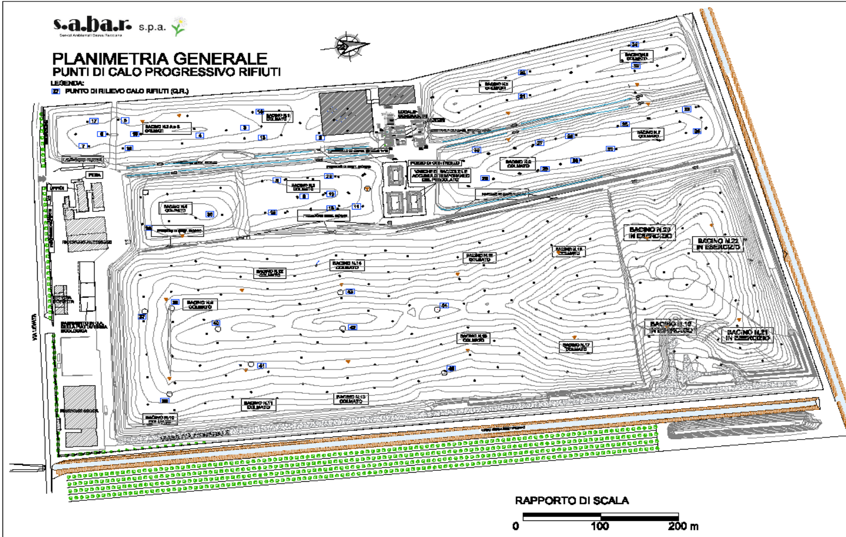
Situazione dei bacini al dicembre 2018
