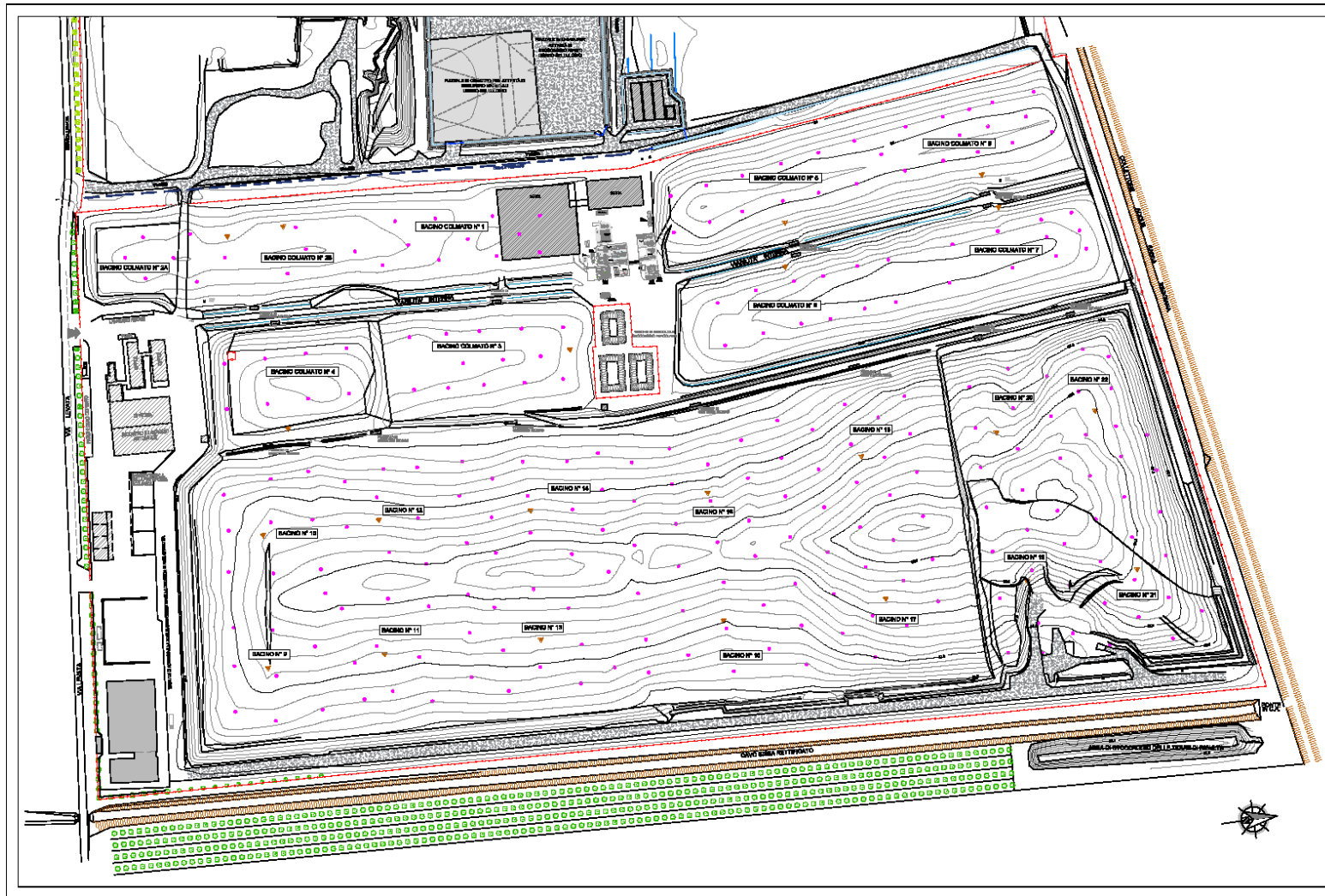
Situazione impiantistica aggiornata al dicembre 2018
