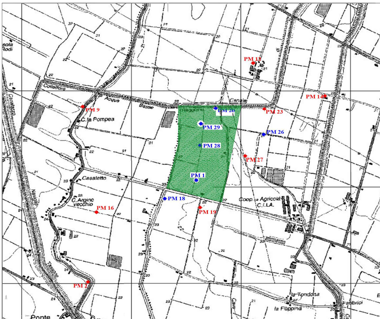
Planimetria con la dislocazione dei Piezometri oggetto del monitoraggio “allargato” di Maggio 2018; in blu i 6 piezometri oggetto del piano di monitoraggio previsto in A.I.A., in rosso piezometri “extra piano”.
