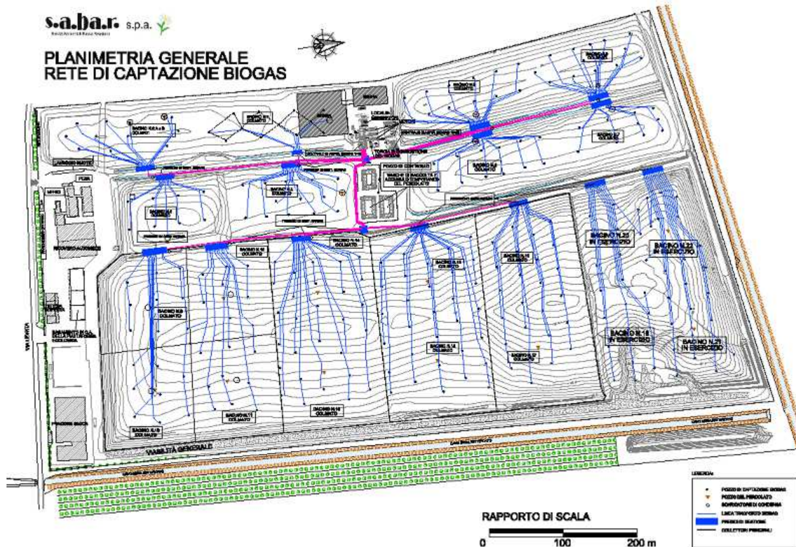
Situazione della rete di captazione del biogas aggiornata al dicembre 2018
