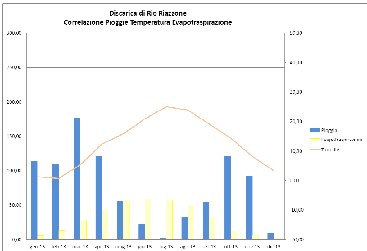
Grafico. n. 6 – Andamento di Temperature medie mensili, piovosità ed evapotraspirazione rilevati presso la Discarica di Rio Riazzone, anno 2013
