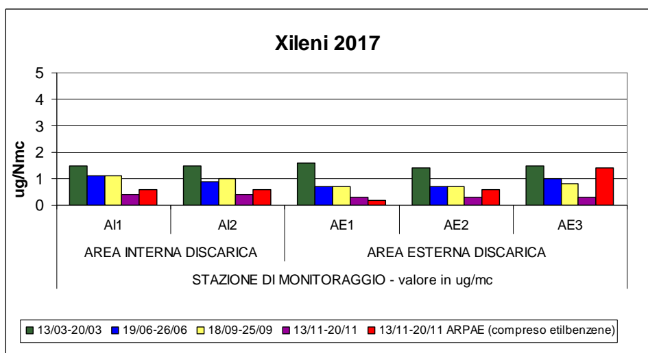
Grafico n. 5 – Andamento Xileni, anno 2017
