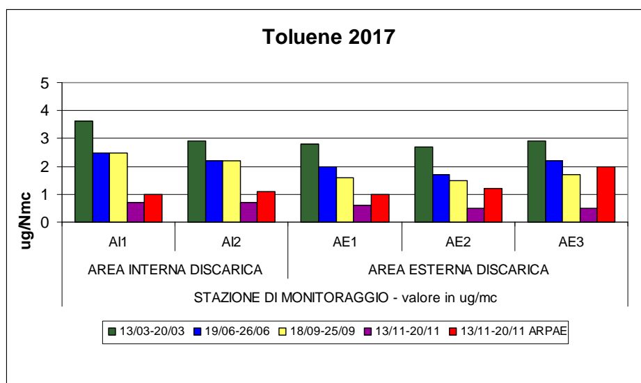
Grafico n. 4 – Andamento Toluene, anno 2017
