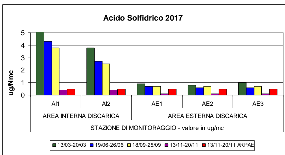
Grafico. n 6 – Andamento Acido Solfidrico, anno 2017
