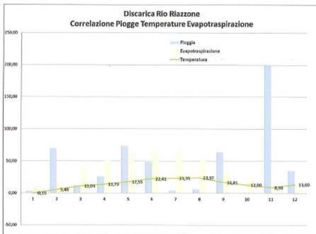
Grafico. n. 7 – Andamento di Temperature medie mensili, piovosità ed evapotraspirazione rilevati presso la Discarica di Rio Riazone, anno 2017
