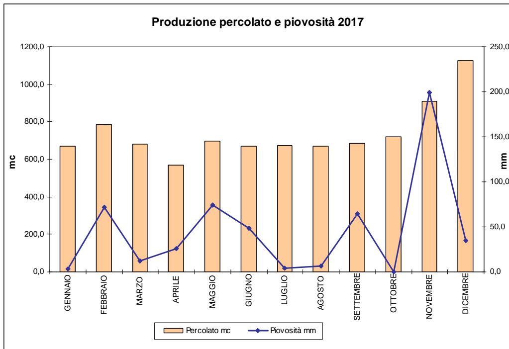
Grafico n. 1 – Andamento della produzione di percolato e piovosità nell'anno 2017
