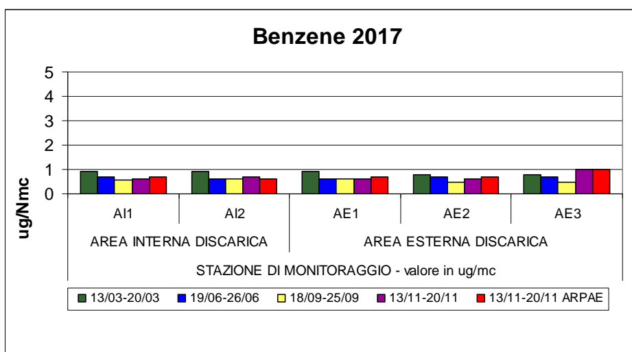
Grafico n. 3 – Andamento Benzene, anno 2017
