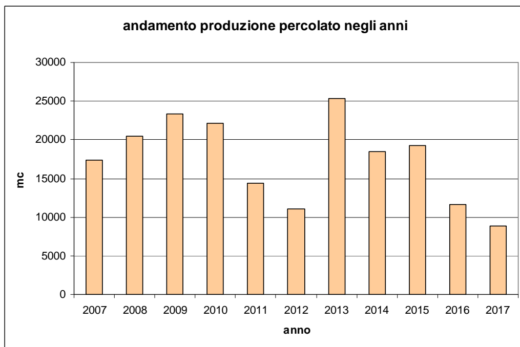
Grafico n. 2 – Andamento della produzione di percolato negli anni
