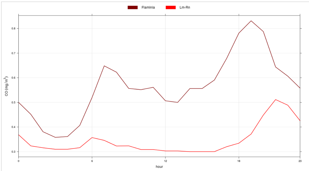
Fig. 3.4.4 - Giorno tipo. Andamento valore medio orario del giorno tipo per il CO (mg/m³) - Campagna Estiva
