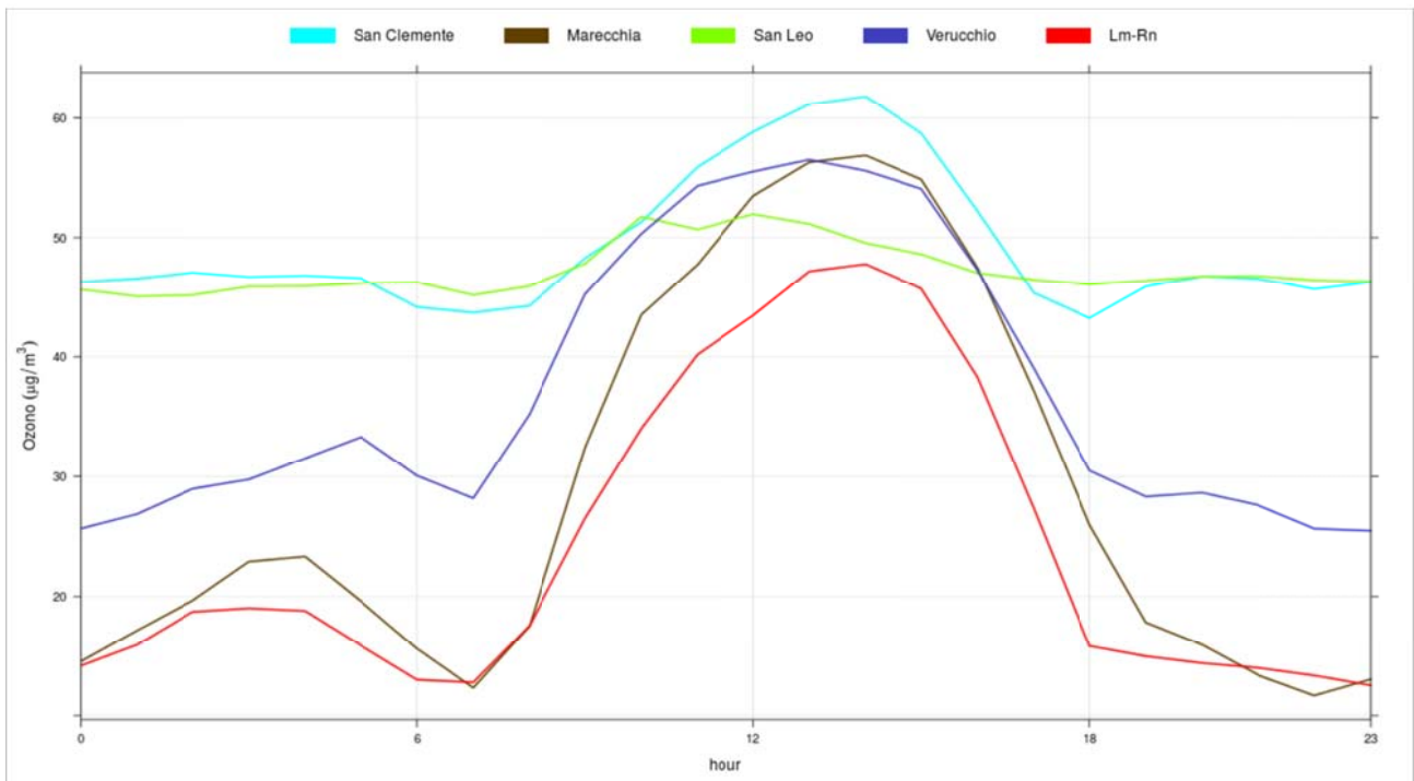
Fig. 3.4.3 - Giorno tipo. Andamento valore medio orario del giorno tipo per per l' Ozono ( \mu\text{g}/\text{m}^3 ) - Campagna Invernale
