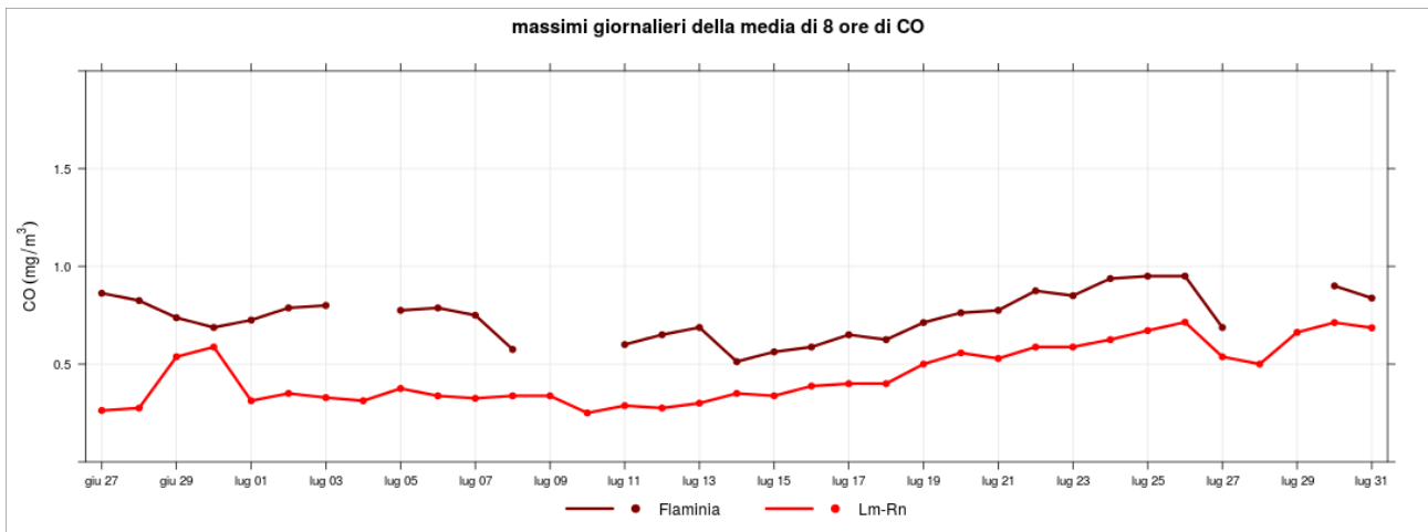
Fig. 3.4.2 - Medie mobili sulle 8 ore registrate con il laboratorio mobile (mg/m³) - Campagna Estiva
