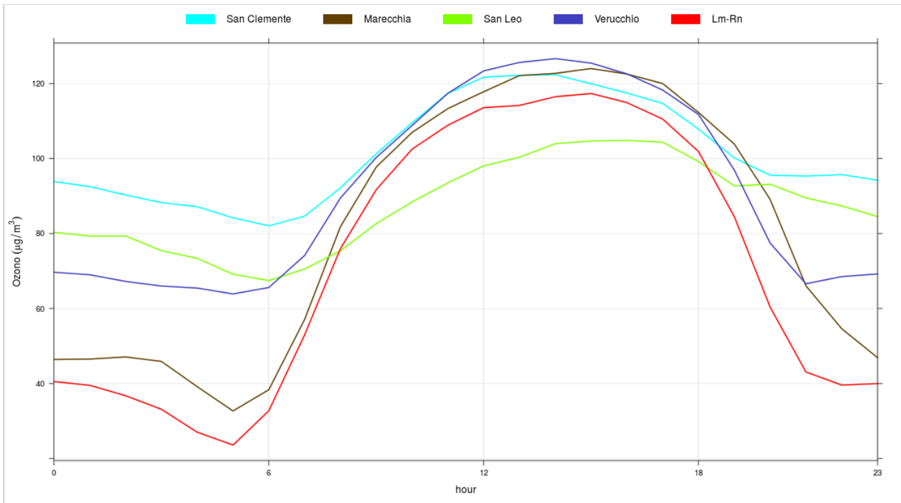
Fig. 3.4.4 - Giorno tipo. Andamento valore medio orario del giorno tipo per per l' Ozono ( \mu\text{g}/\text{m}^3 ) - Campagna Estiva
