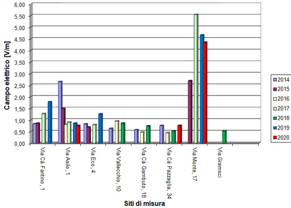
Valori massimi di campo elettrico riferiti ad ogni sito oggetto di indagine per gli anni 2014 - 2015 - 2016 - 2017 - 2018 - 2019 - 2020
