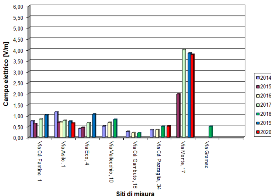
Valori medi di campo elettrico riferiti ad ogni sito oggetto di indagine per gli anni 2014 - 2015 - 2016 - 2017 - 2018 - 2019 - 2020
