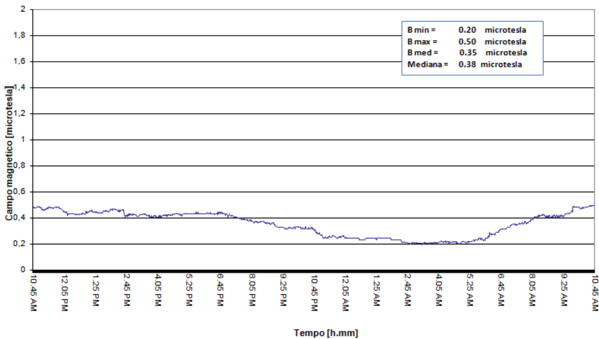
Fig. n. 2 - Andamento del campo magnetico dal 6 al 7 febbraio 2018
