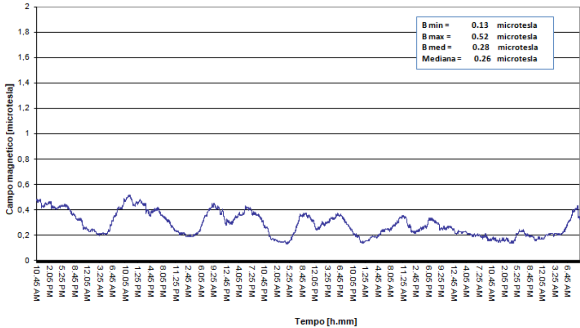
Fig. n. 1 - Andamento del campo magnetico dal 6 al 12 febbraio 2018
