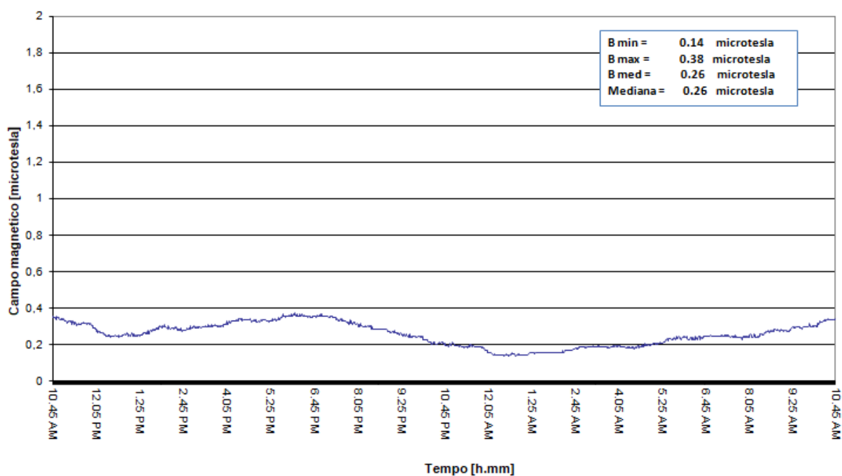
Fig. n. 5 - Andamento del campo magnetico dal 09 al 10 febbraio 2018
