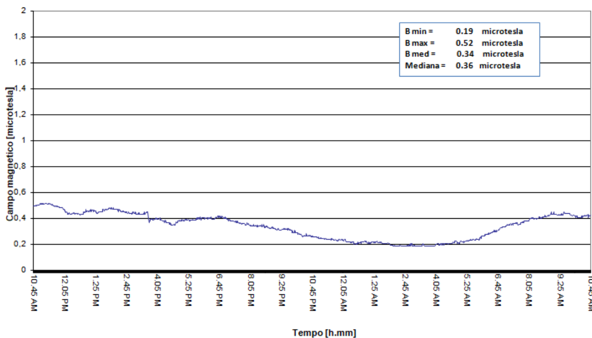
Fig. n. 3 - Andamento del campo magnetico dal 7 all' 8 febbraio 2018
