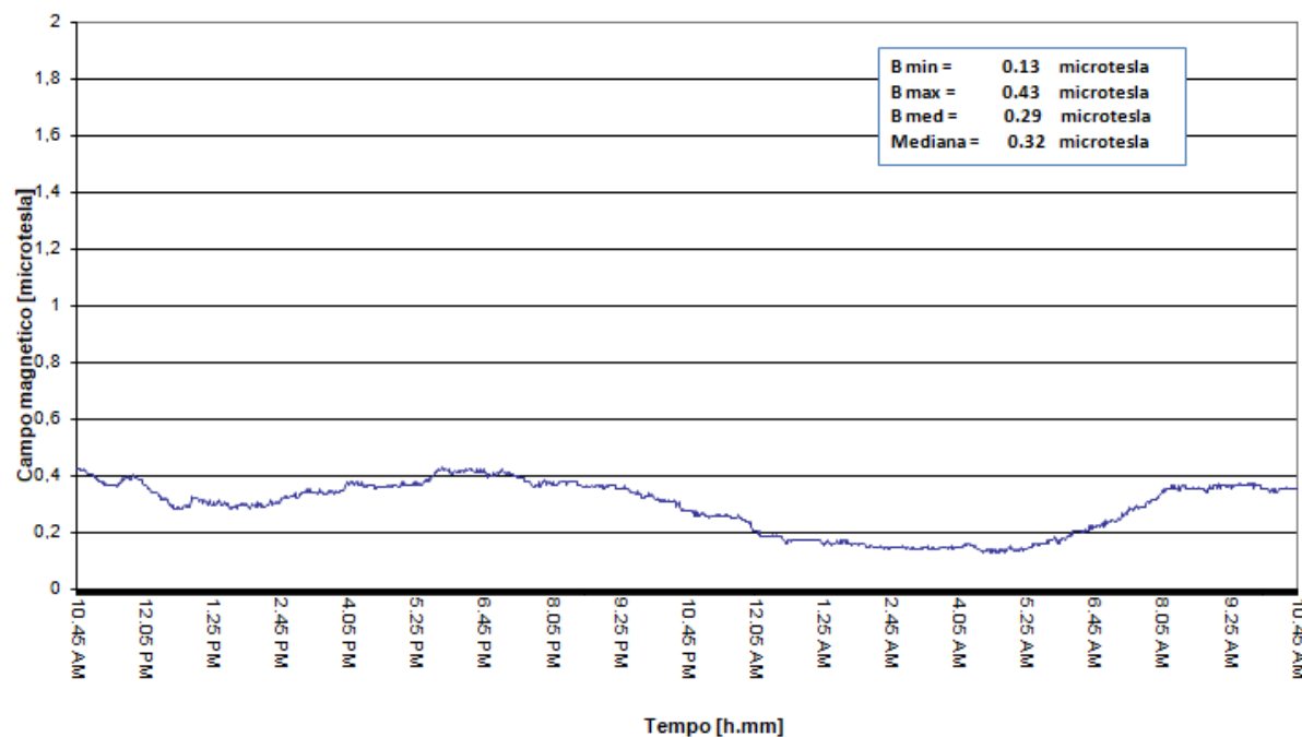
Fig. n. 4 - Andamento del campo magnetico dall'8 al 9 febbraio 2018
