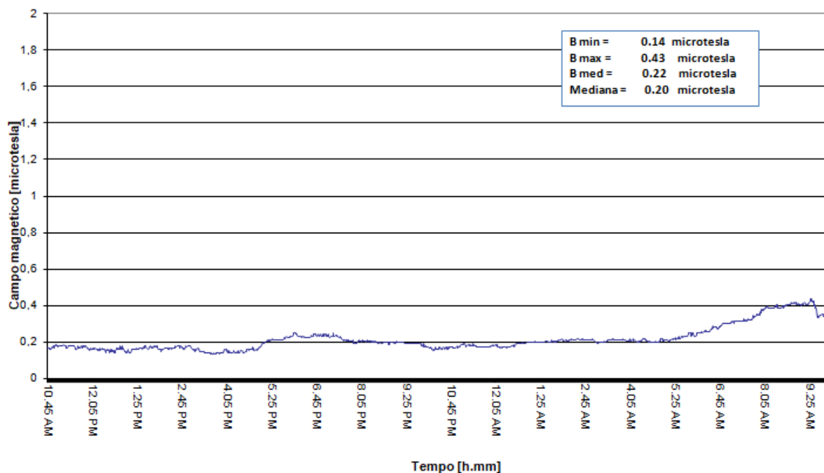
Fig. n. 7 - Andamento del campo magnetico dal 11 al 12 febbraio 2018
