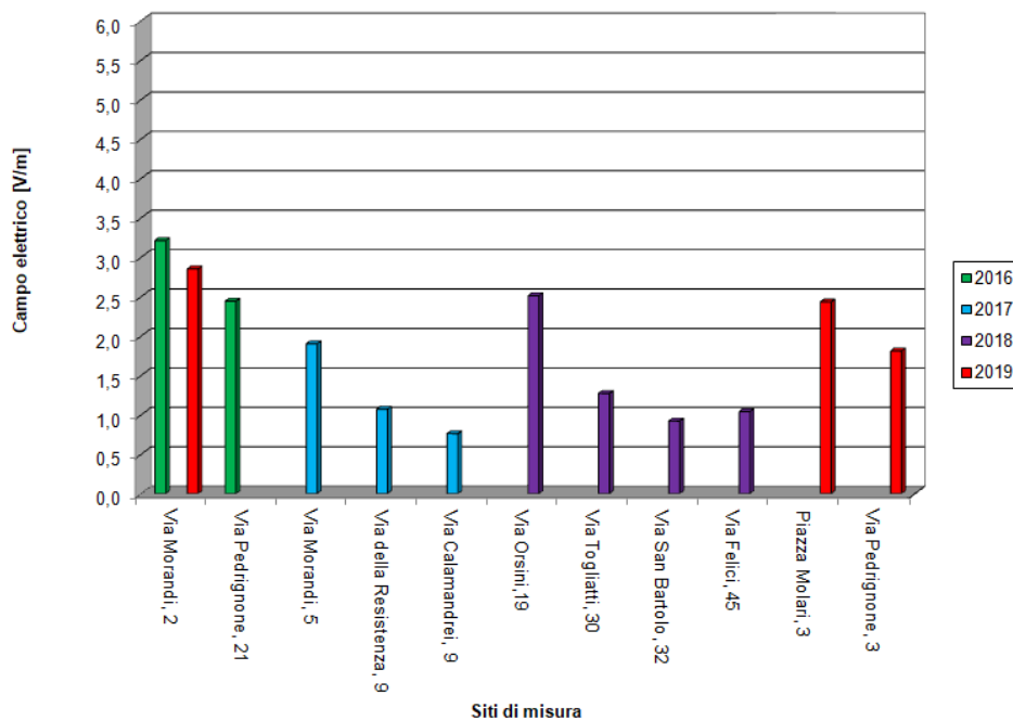
Valori massimi di campo elettrico riferiti ad ogni sito oggetto di indagine per gli anni 2016 - 2017 - 2018 - 2019
