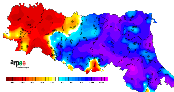
Anomalia del Bilancio Idroclimatico (mm) dal 01/01/2023 al 24/09/2023
