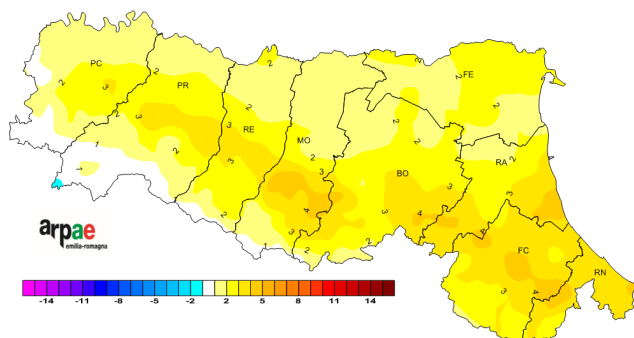
Anomalia delle Temperature Massime settimanali (°C) dal 18/09/2023 al 24/09/2023
