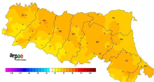
Anomalia della Temperature Medie settimanali (°C) dal 25/12/2023 al 31/12/2023
