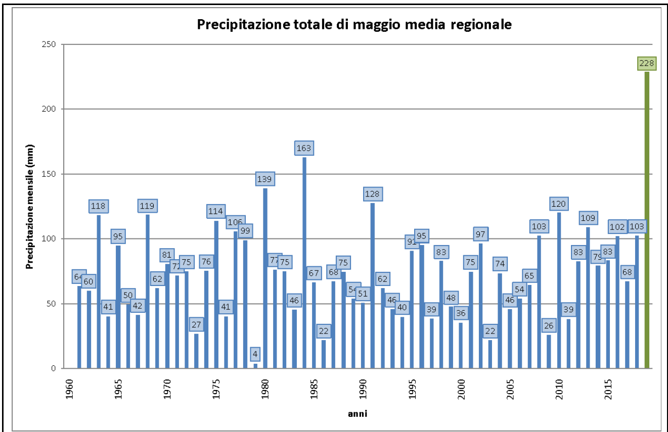
Fig.2: Serie temporale della precipitazione totale di maggio mediata sull'Emilia-Romagna(data-set Eraclito )
