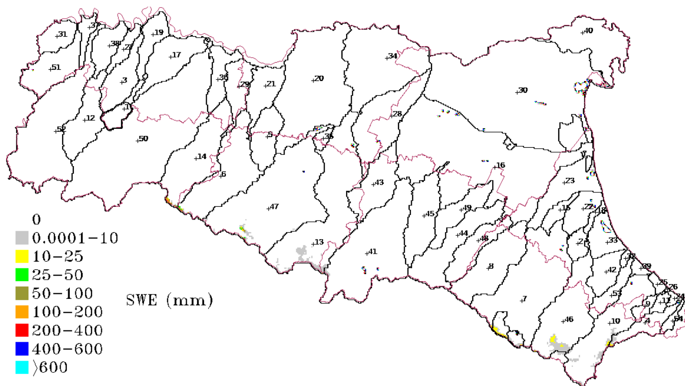
Fig. 2 – Equivalente in acqua della neve (SWE – mm): integrazione dati da modello e satellite
