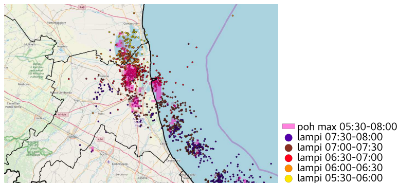
Figura 29. Probabilità di grandine superiore al 99% nell'intervallo temporale tra le 05:30 UTC e le 08:00 UTC del 10/07/2019, in fucsia, sovrapposta alle fulminazioni rilevate dalla rete LAMPINET sulle province di Ferrara e Ravenna.
