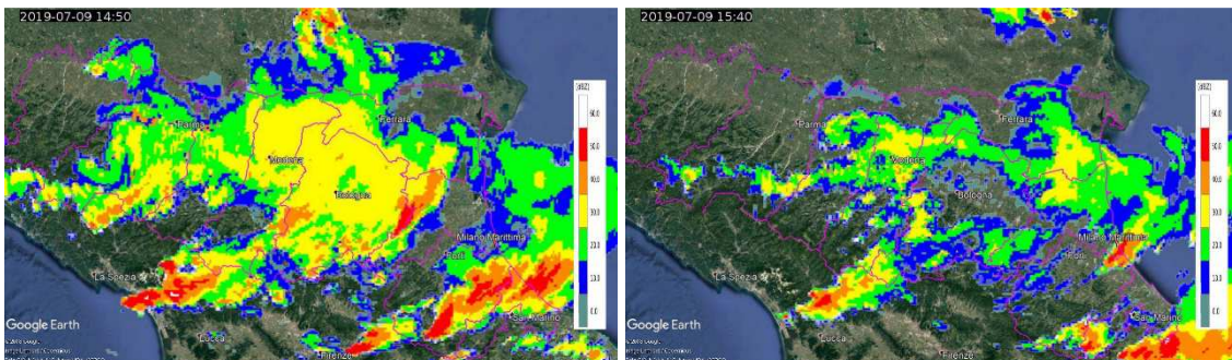
Figura 16. Mappe di riflettività del 09/07/2019 alle 14:50 UTC (a sinistra) e alle ore 15:40 UTC (a destra).
