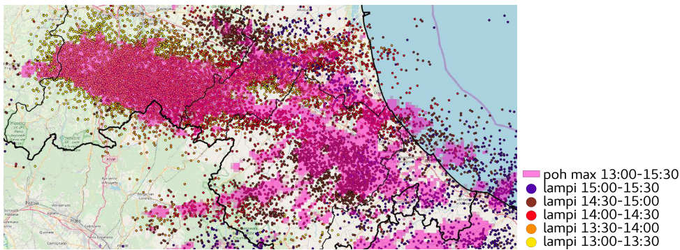
Figura 28. Probabilità di grandine superiore al 99% nell'intervallo temporale tra le 13:00 UTC e le 15:30 UTC del 09/07/2019, in fucsia, sovrapposta alle fulminazioni rilevate dalla rete LAMPINET sulle province di Bologna, Ravenna, Forlì-Cesena e Rimini.
