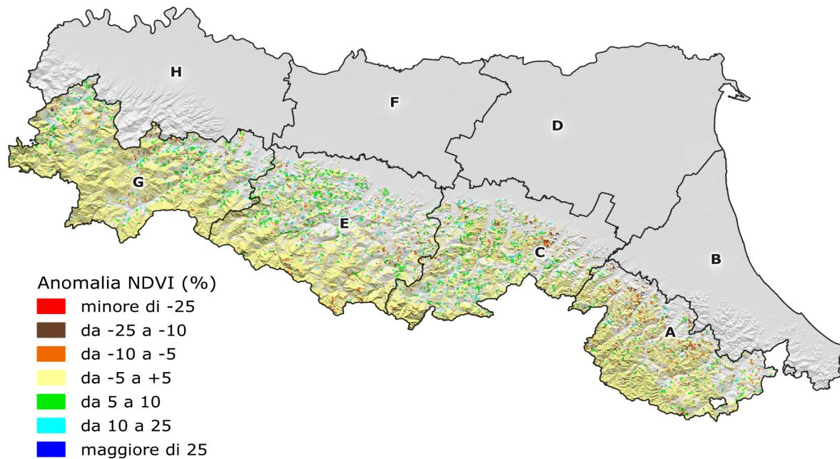
Figura 1 - Anomalia di NDVI sulle macroaree a elevata copertura forestale rispetto alla serie 2016-2023
