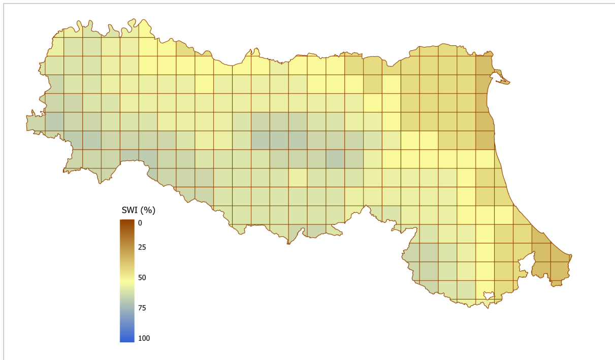
Figura 7 - Soil Water Index sul territorio regionale, risoluzione 12 km. La mappa rappresenta i valori medi di SWI sul periodo di riferimento.
