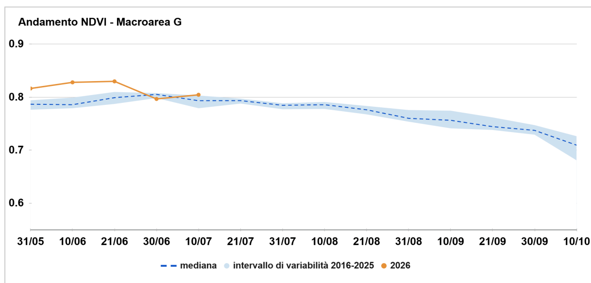
Figura 5 - Macroarea G: il grafico mostra l'andamento della mediana dell'indice NDVI dell'anno in corso (linea arancione) confrontato con la mediana del periodo 2016-2025 (linea tratteggiata) e l'intervallo di variabilità (fascia azzurra), delimitato in alto dal 75° e in basso dal 25° percentile.
