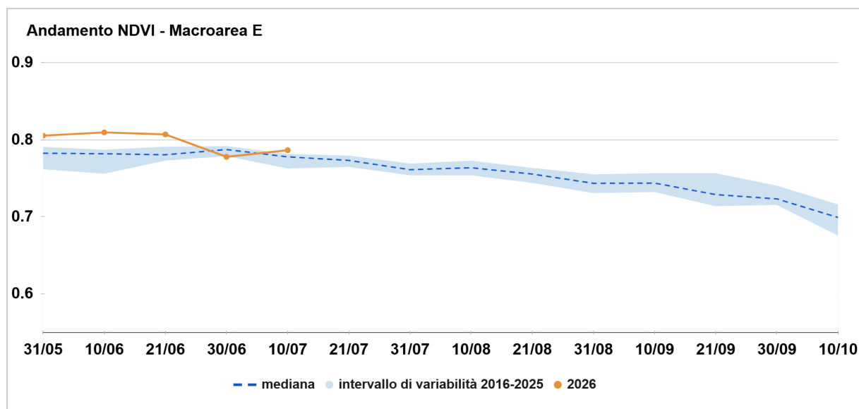
Figura 4 - Macroarea E: il grafico mostra l'andamento della mediana dell'indice NDVI dell'anno in corso (linea arancione) confrontato con la mediana del periodo 2016-2025 (linea tratteggiata) e l'intervallo di variabilità (fascia azzurra), delimitato in alto dal 75° e in basso dal 25° percentile.
