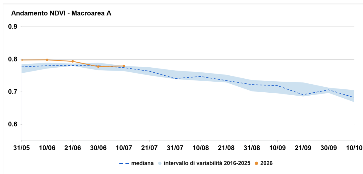
Figura 2 - Macroarea A: il grafico mostra l'andamento della mediana dell'indice NDVI dell'anno in corso (linea arancione) confrontato con la mediana del periodo 2016-2025 (linea tratteggiata) e l'intervallo di variabilità (fascia azzurra), delimitato in alto dal 75° e in basso dal 25° percentile.
