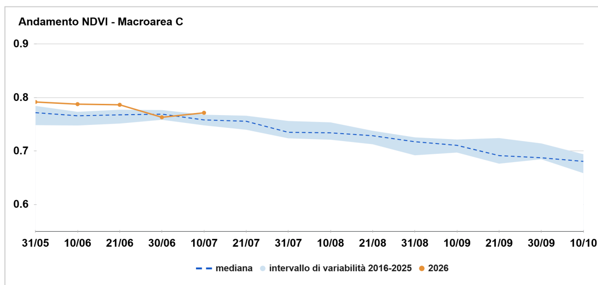
Figura 3 - Macroarea C: il grafico mostra l'andamento della mediana dell'indice NDVI dell'anno in corso (linea arancione) confrontato con la mediana del periodo 2016-2025 (linea tratteggiata) e l'intervallo di variabilità (fascia azzurra), delimitato in alto dal 75° e in basso dal 25° percentile.
