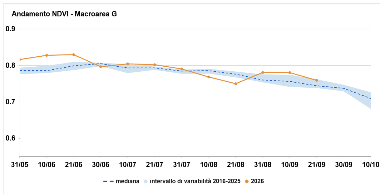
Figura 5 - Macroarea G: il grafico mostra l'andamento della mediana dell'indice NDVI dell'anno in corso (linea arancione) confrontato con la mediana del periodo 2016-2025 (linea tratteggiata) e l'intervallo di variabilità (fascia azzurra), delimitato in alto dal 75° e in basso dal 25° percentile.
