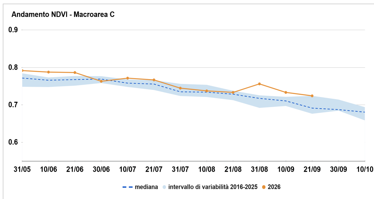
Figura 3 - Macroarea C: il grafico mostra l'andamento della mediana dell'indice NDVI dell'anno in corso (linea arancione) confrontato con la mediana del periodo 2016-2025 (linea tratteggiata) e l'intervallo di variabilità (fascia azzurra), delimitato in alto dal 75° e in basso dal 25° percentile.
