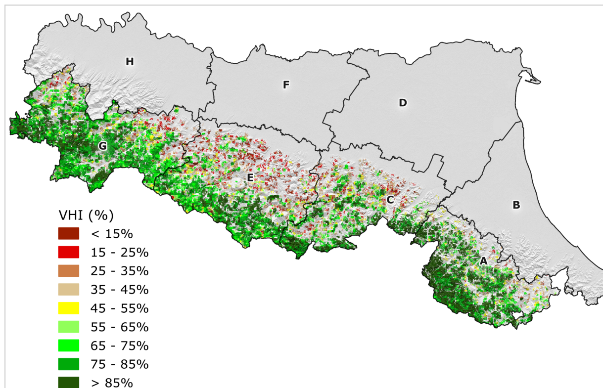
Figura 6 - Indice VHI sulle macroaree a elevata copertura forestale.
