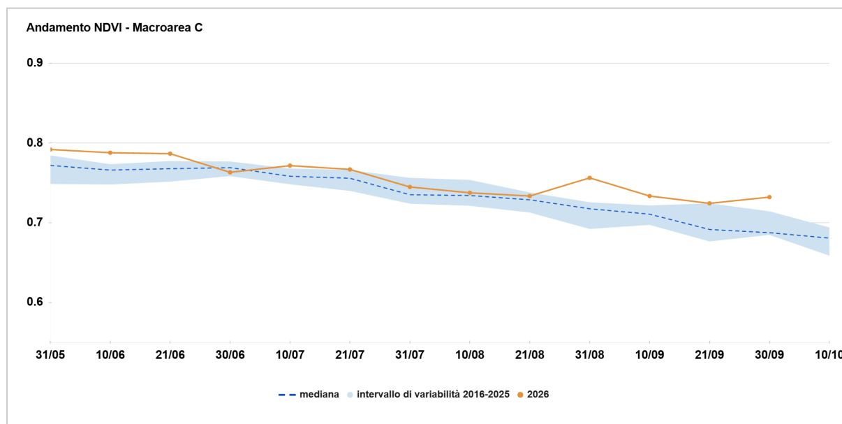
Figura 3 - Macroarea C: il grafico mostra l'andamento della mediana dell'indice NDVI dell'anno in corso (linea arancione) confrontato con la mediana del periodo 2016-2025 (linea tratteggiata) e l'intervallo di variabilità (fascia azzurra), delimitato in alto dal 75° e in basso dal 25° percentile.
