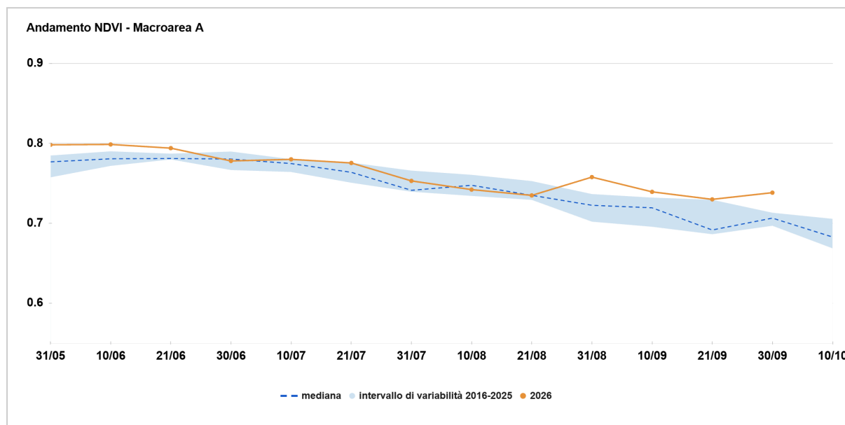
Figura 2 - Macroarea A: il grafico mostra l'andamento della mediana dell'indice NDVI dell'anno in corso (linea arancione) confrontato con la mediana del periodo 2016-2025 (linea tratteggiata) e l'intervallo di variabilità (fascia azzurra), delimitato in alto dal 75° e in basso dal 25° percentile.
