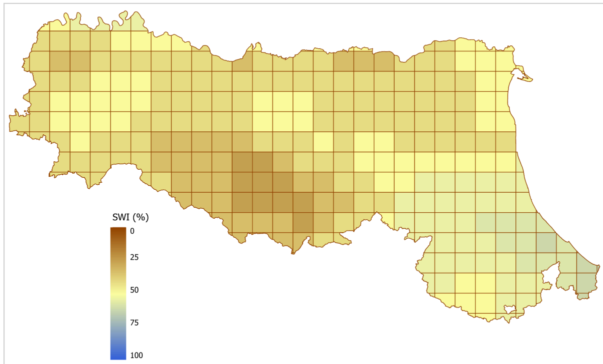
Figura 7 - Soil Water Index sul territorio regionale, risoluzione 12 km. La mappa rappresenta i valori medi di SWI sul periodo di riferimento.
