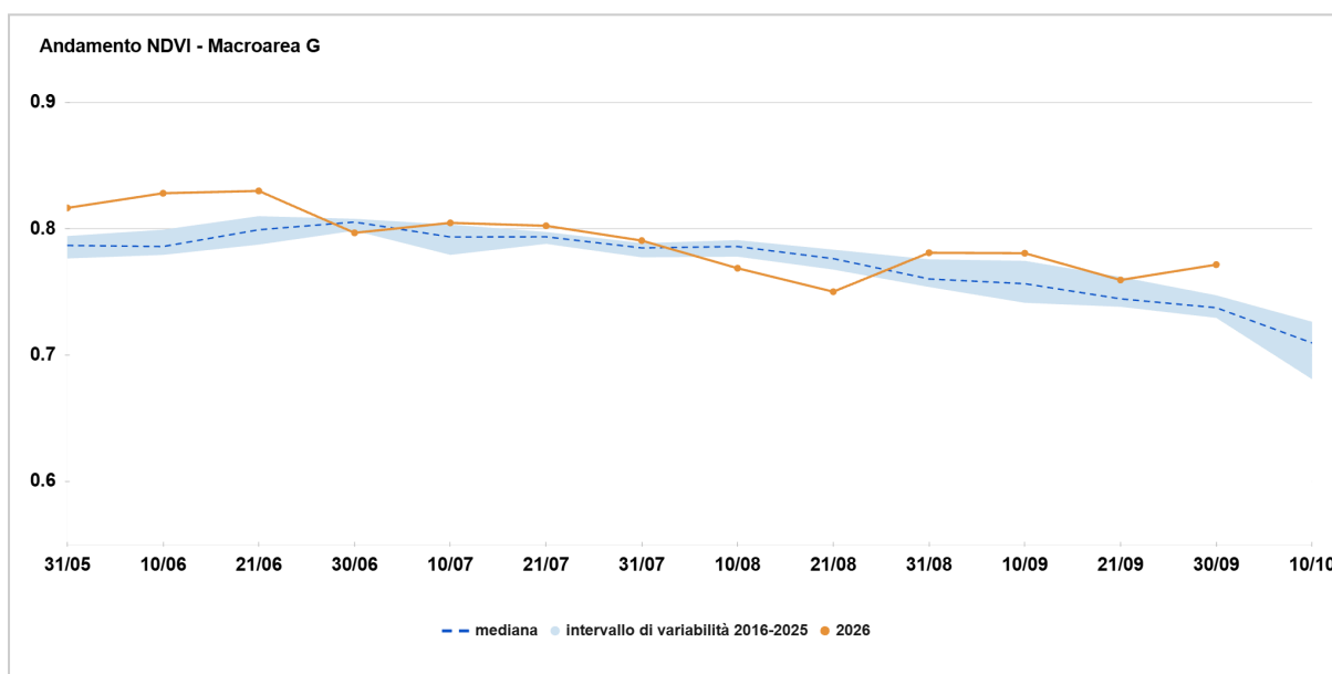
Figura 5 - Macroarea G: il grafico mostra l'andamento della mediana dell'indice NDVI dell'anno in corso (linea arancione) confrontato con la mediana del periodo 2016-2025 (linea tratteggiata) e l'intervallo di variabilità (fascia azzurra), delimitato in alto dal 75° e in basso dal 25° percentile.
