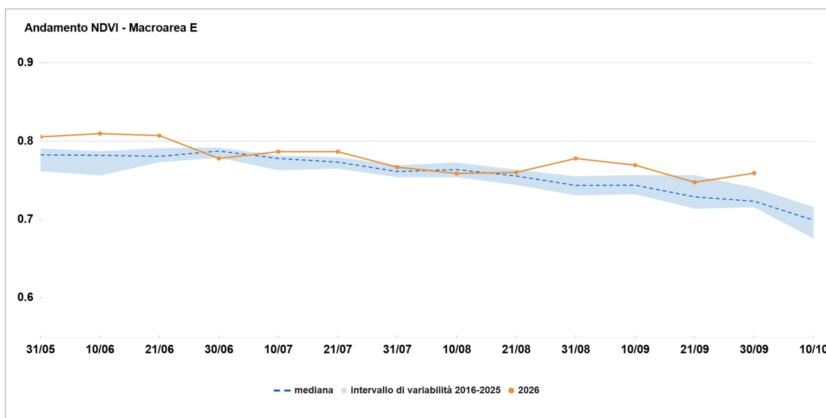
Figura 4 - Macroarea E: il grafico mostra l'andamento della mediana dell'indice NDVI dell'anno in corso (linea arancione) confrontato con la mediana del periodo 2016-2025 (linea tratteggiata) e l'intervallo di variabilità (fascia azzurra), delimitato in alto dal 75° e in basso dal 25° percentile.
