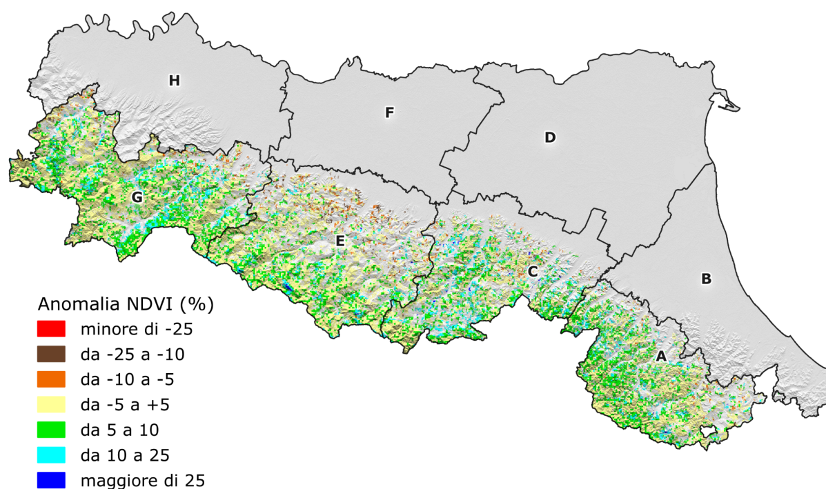
Figura 1 - Anomalia di NDVI sulle macroaree a elevata copertura forestale rispetto alla serie 2016-2025
